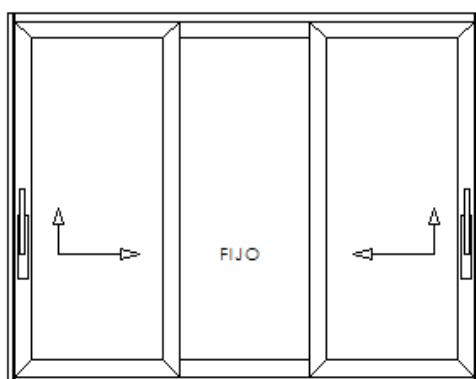
Puerta Elevable 2 Hojas + 1 Fijo 400-3
