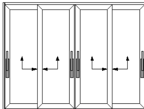
Puerta Elevable 4 Hojas 200-5
